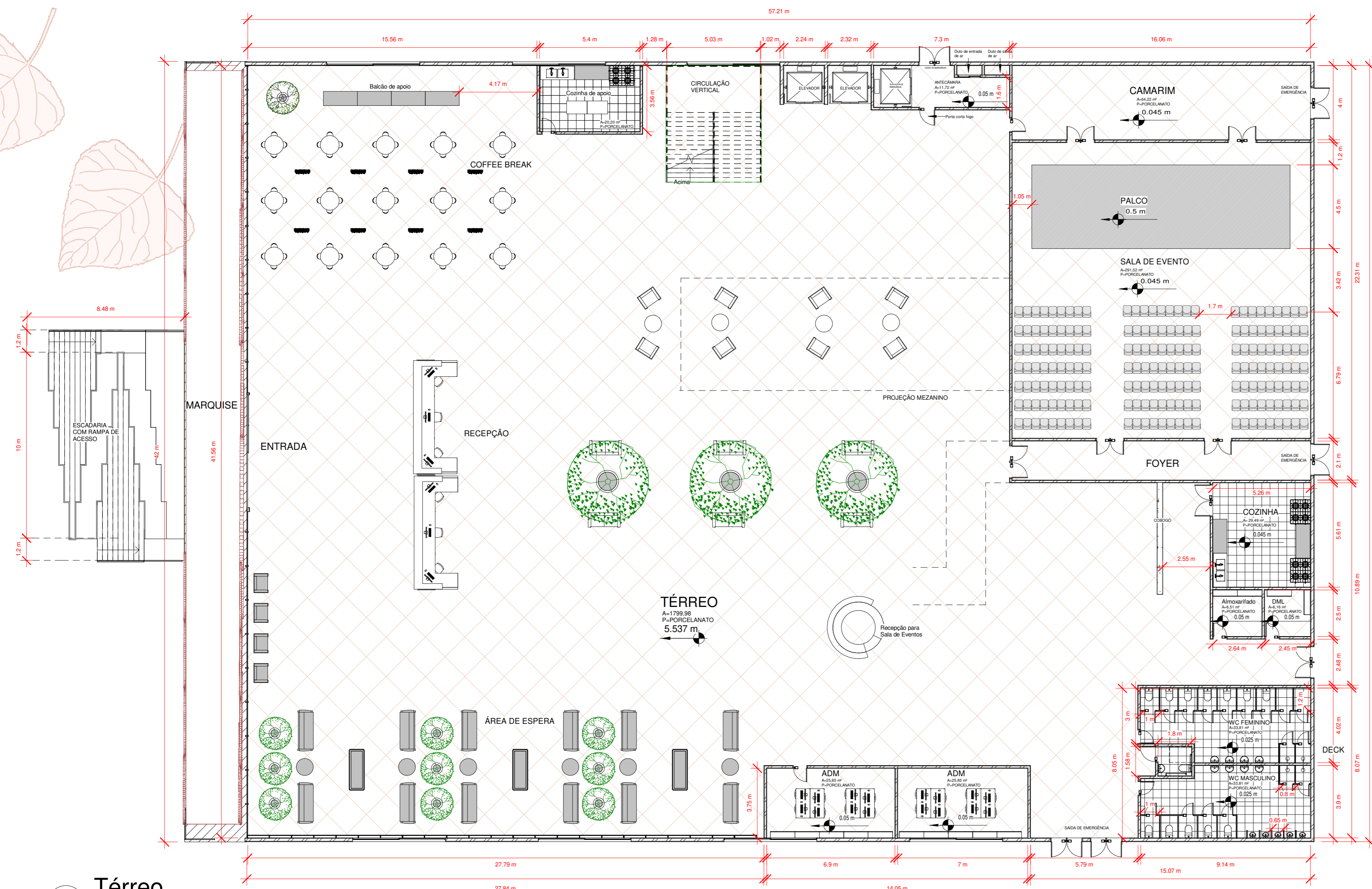
1 Térreo 1 : 150
