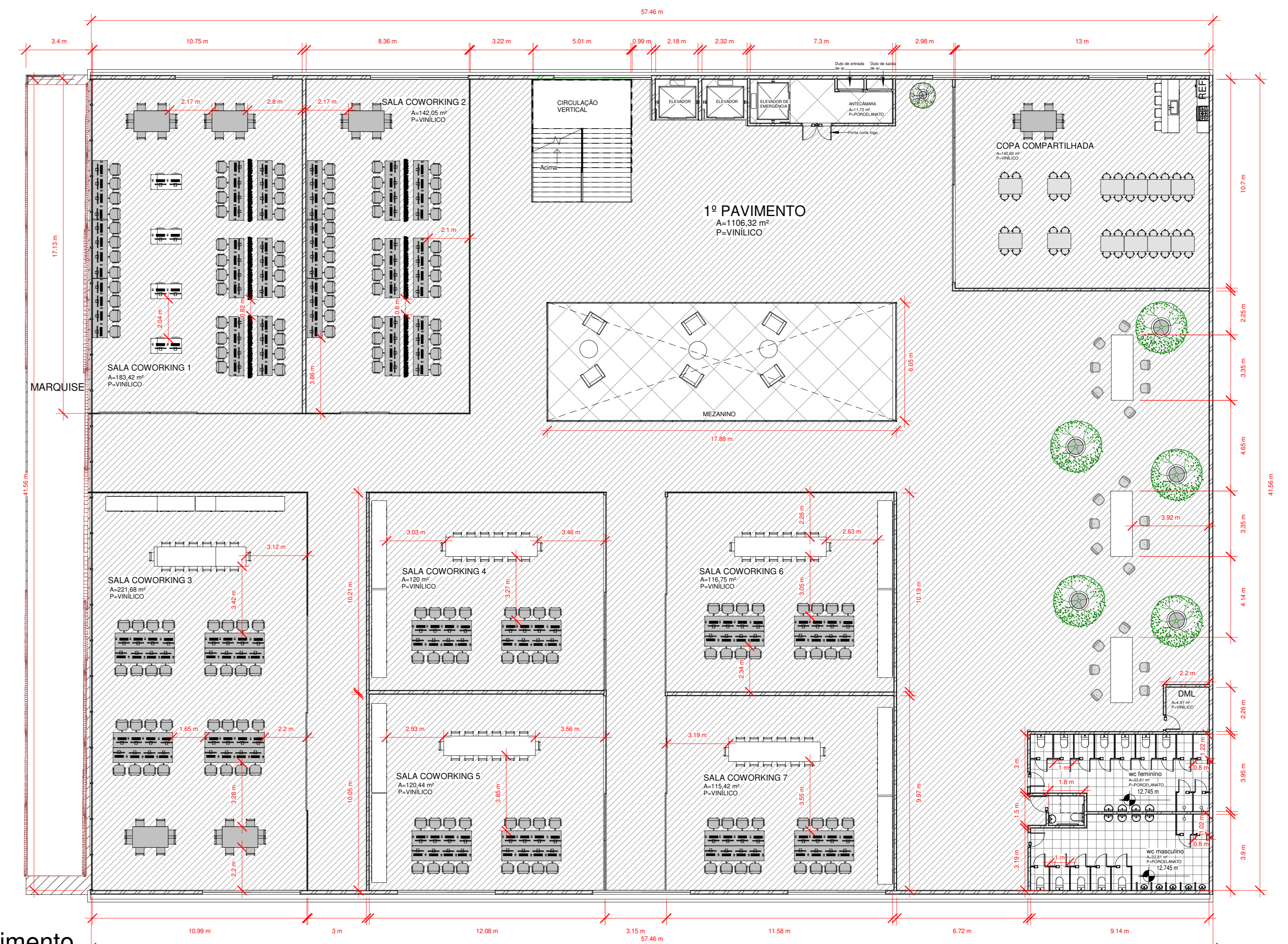
2 1º Pavimento 1 : 150
