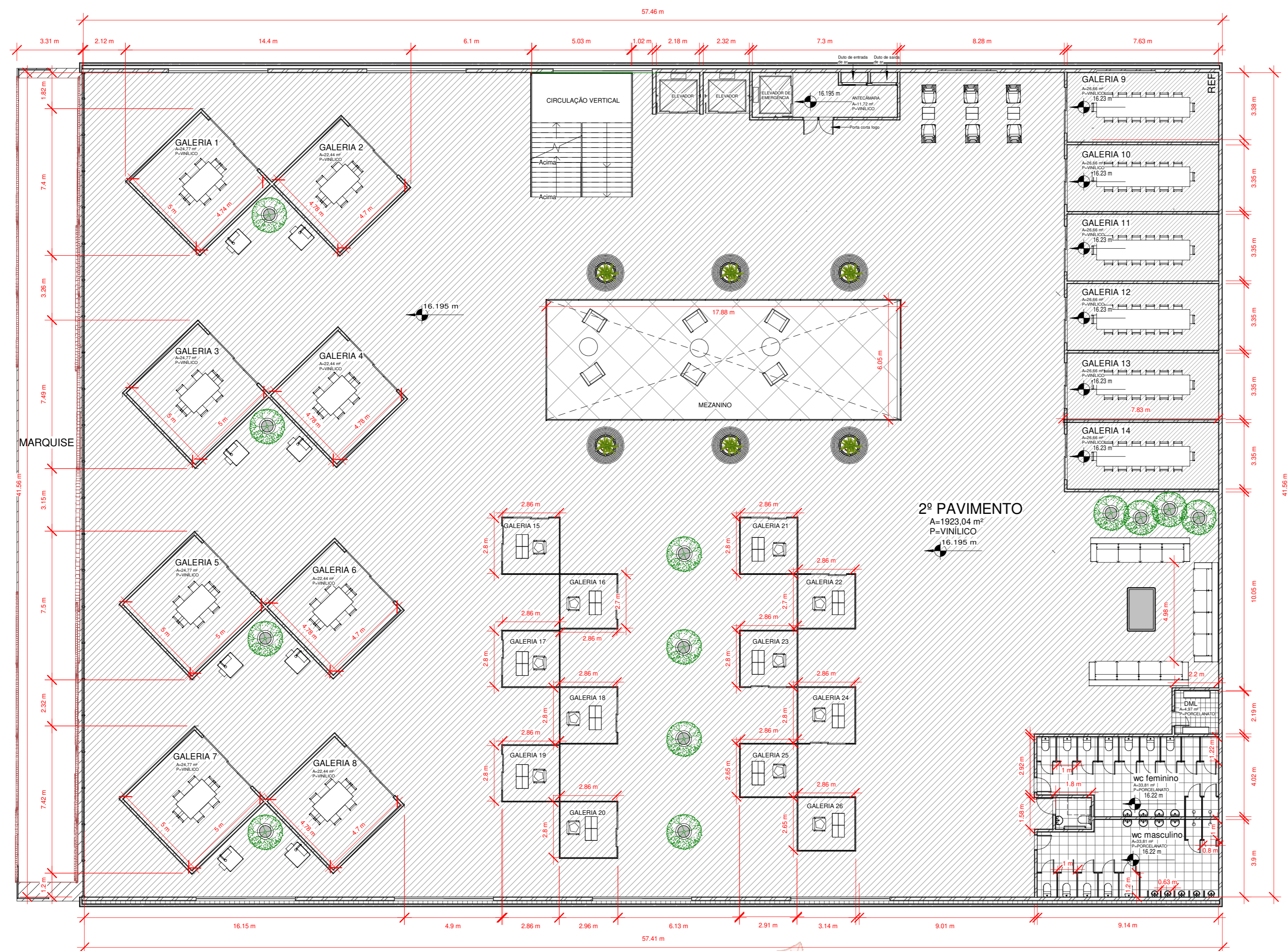
3 2º Pavimento 1 : 150
