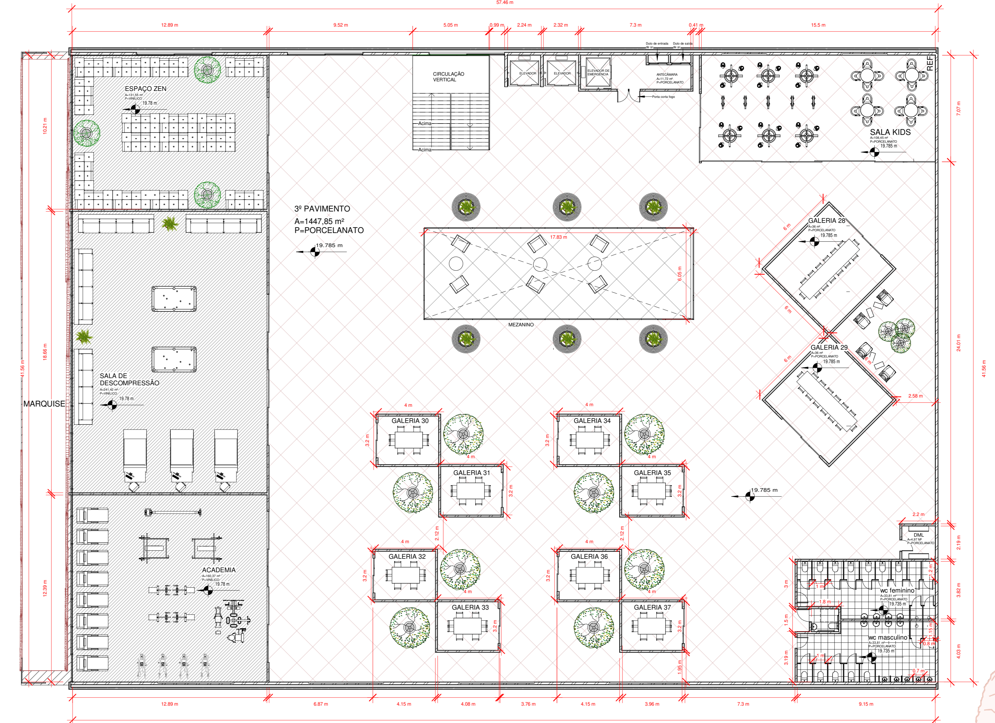
4 3º Pavimento 1 : 150
