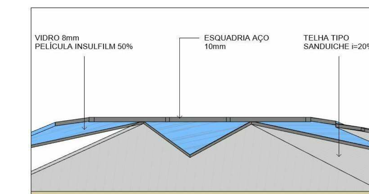
IMAGEM ESTRUTURA VIDRO ESPAÇO BEM ESTAR
