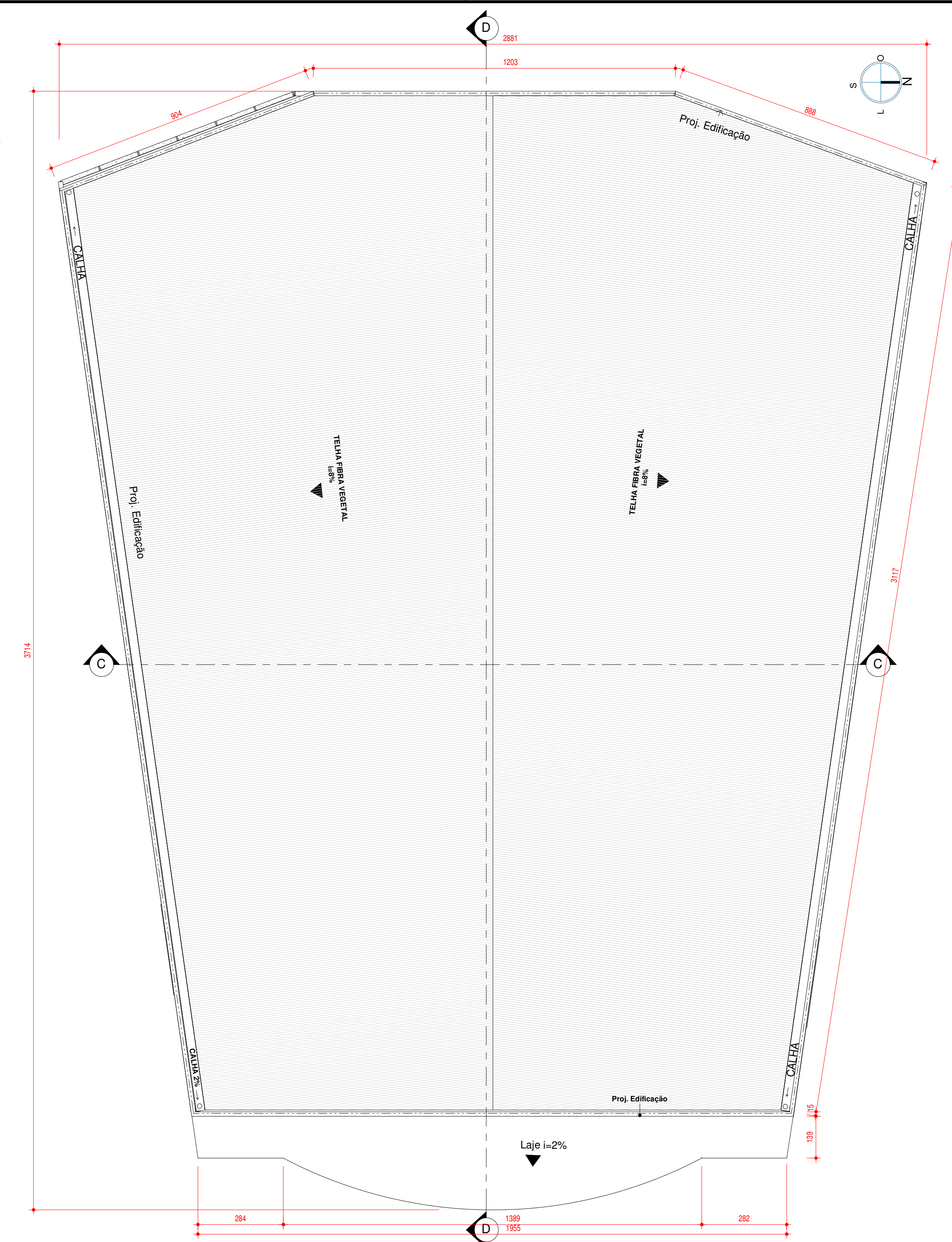
PLANTA BAIXA COLUMBÁRIO ESC:1/100
