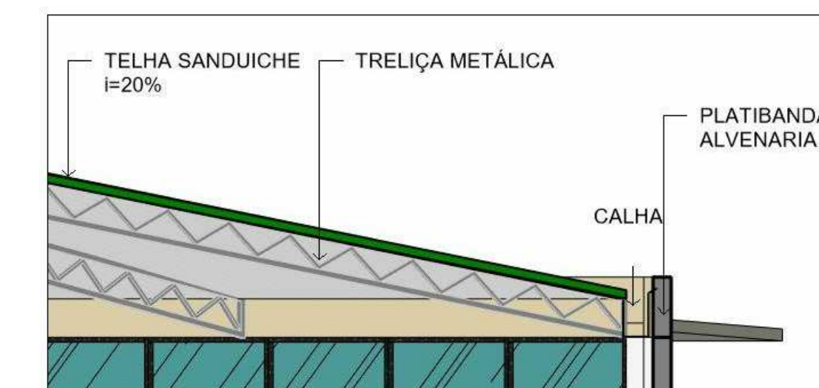
IMAGEM ESTRUTURA TELHADO ESPAÇO BEM ESTAR
