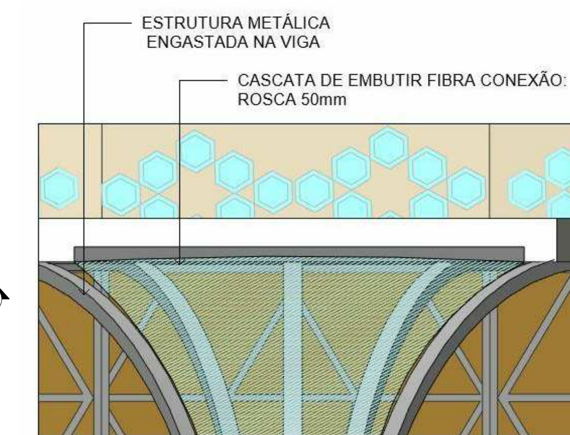
IMAGEM DETALHE CASCATA FIBRA DE IMBUTIR
