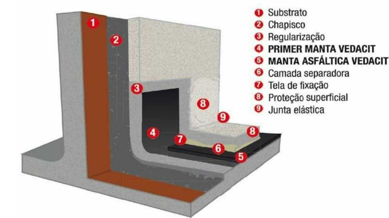
IMAGEM DETALHE LAJE IMPERMEABILIZADA AUDITÓRIO
