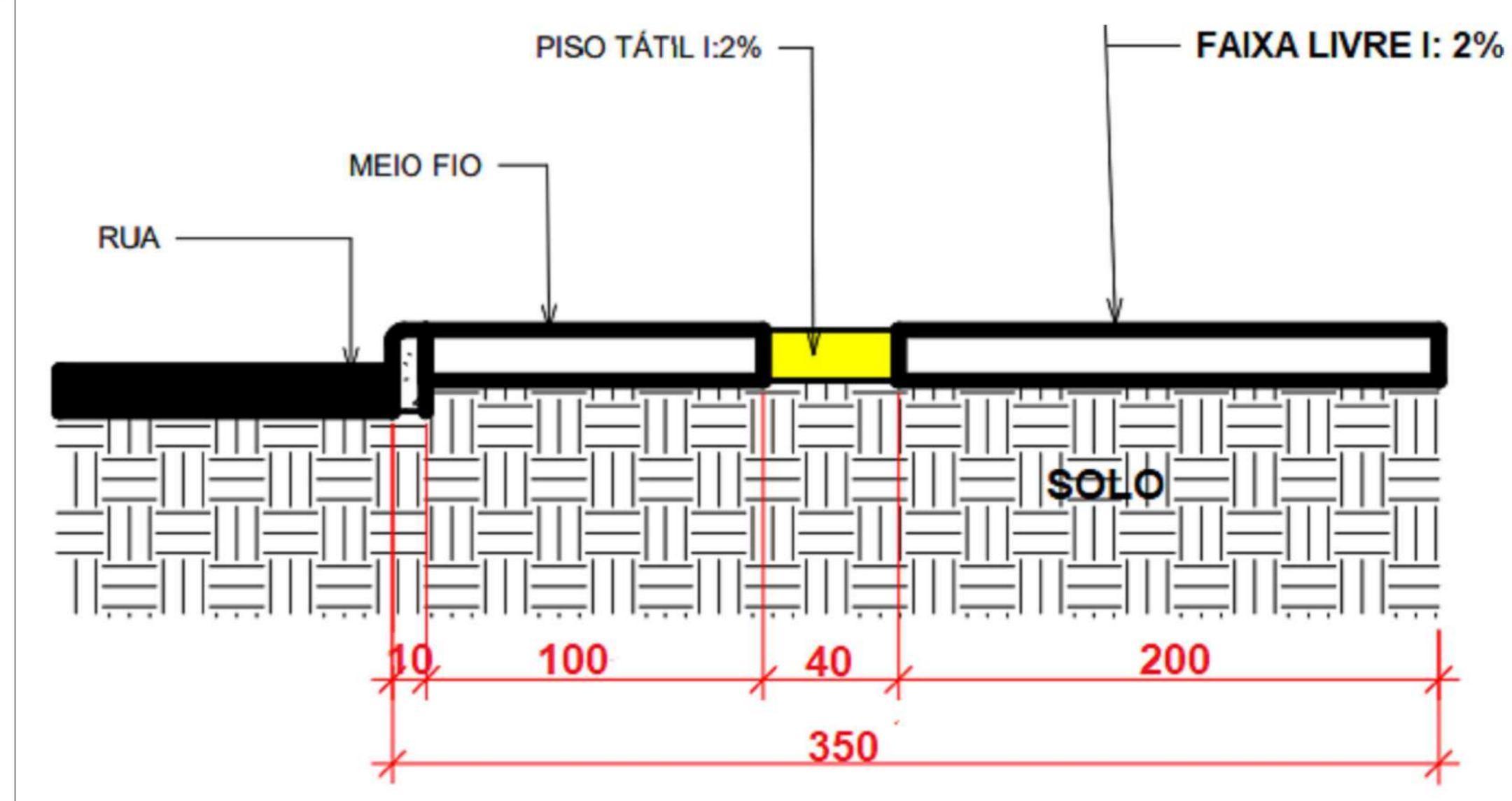
DETALHAMENTO - CALÇADA
