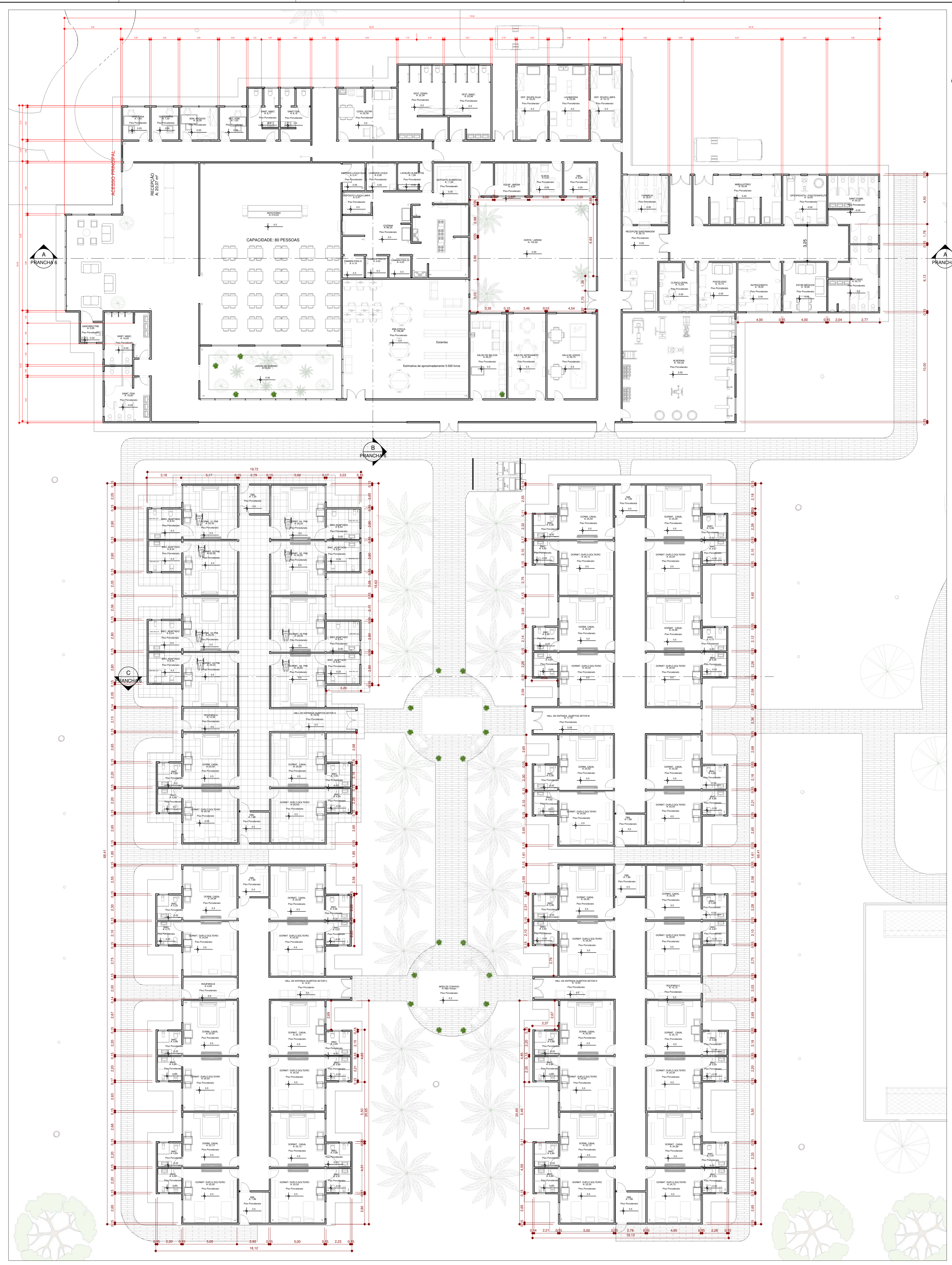
PLANTA BAIXA TÉRREO 1 : 150
