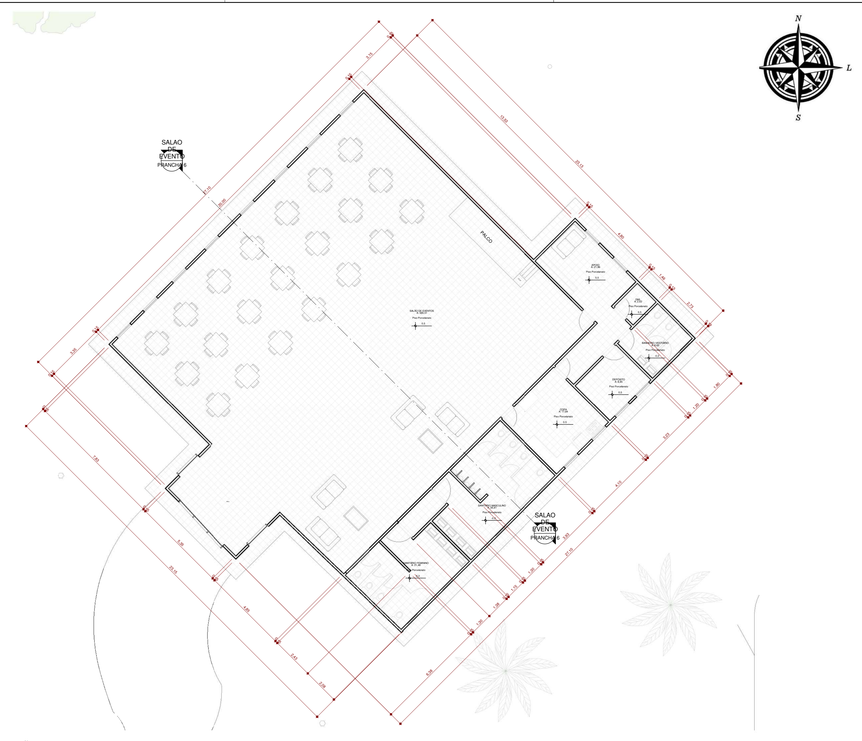
SALÃO DE EVENTOS 1 : 100
