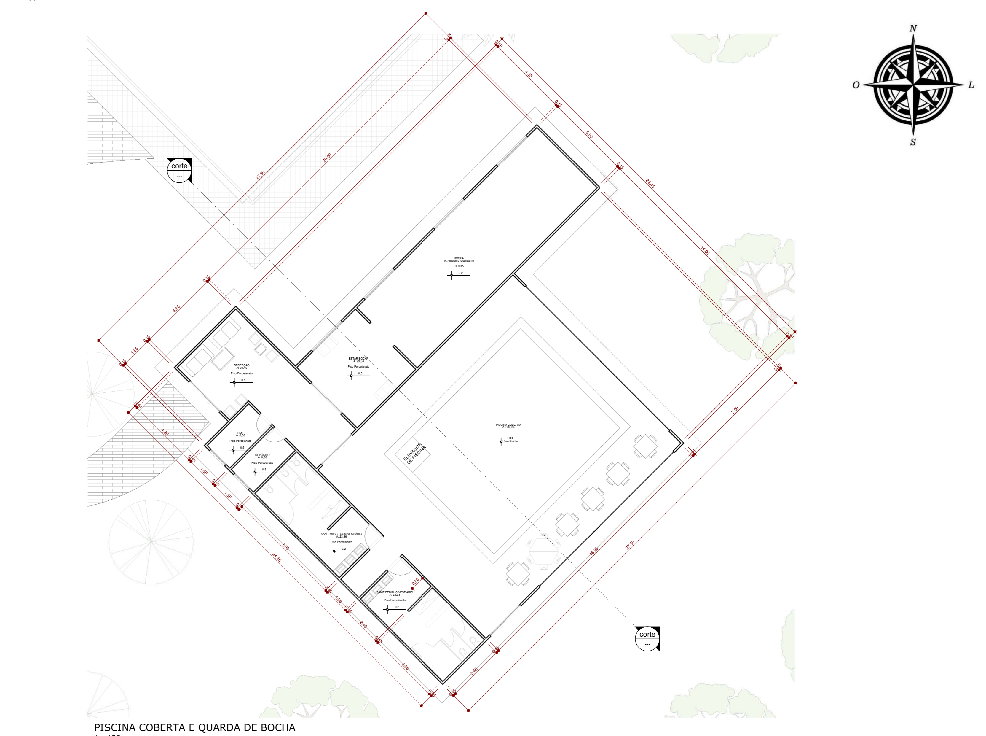
PISCINA COBERTA E GUARDA DE BOCHA 1 : 120
