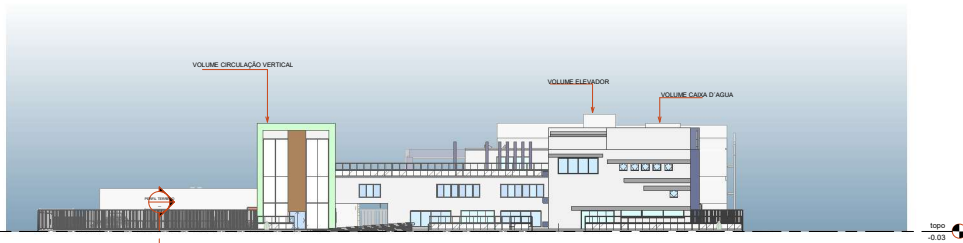
6 Norte 1:200
