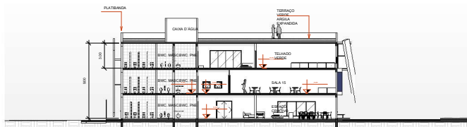
2 CORTE A2 1:150
