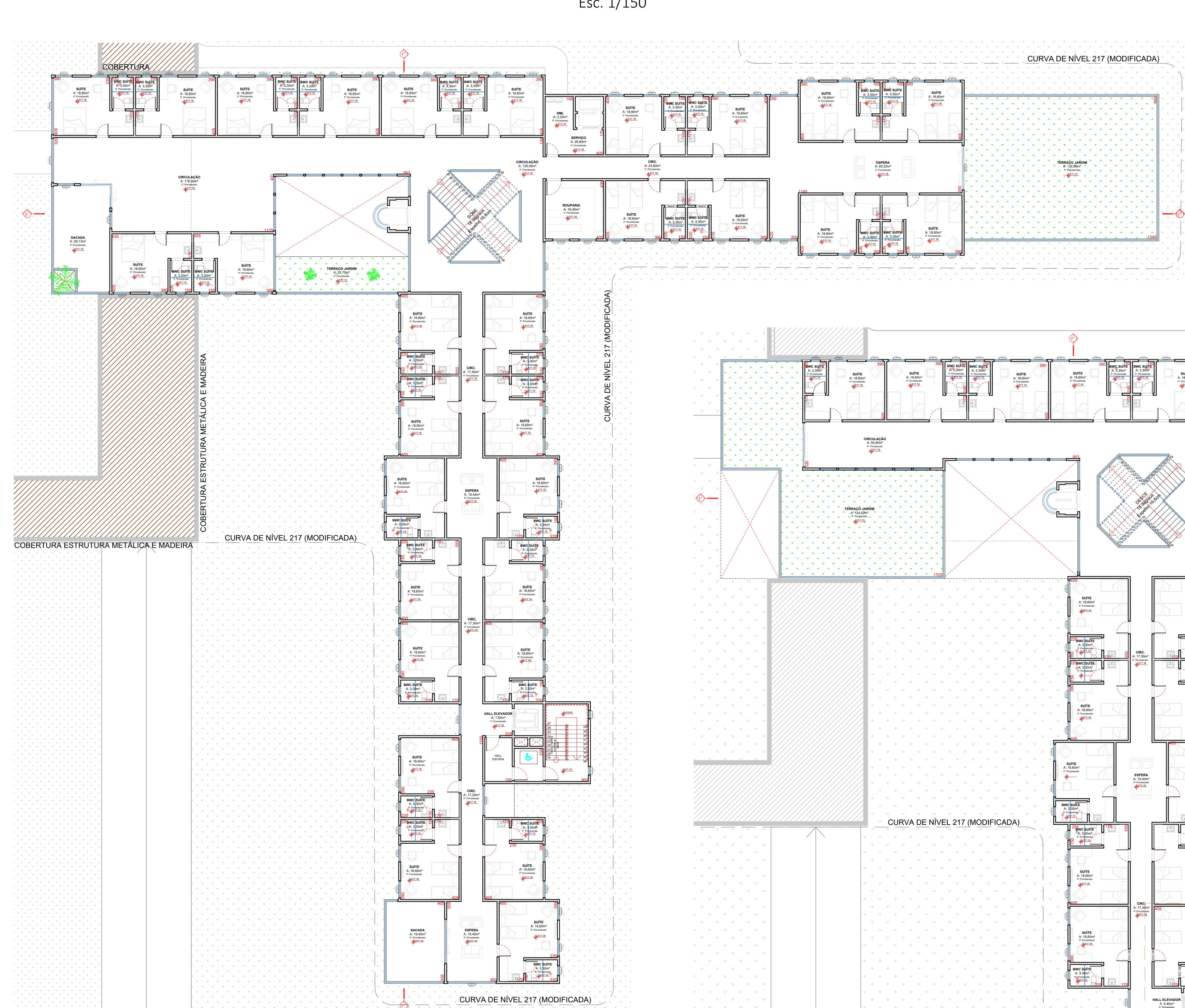
PLANTA BAIXA SETOR DORMITÓRIOS - 1º PAVIMENTO Esc. 1/150
