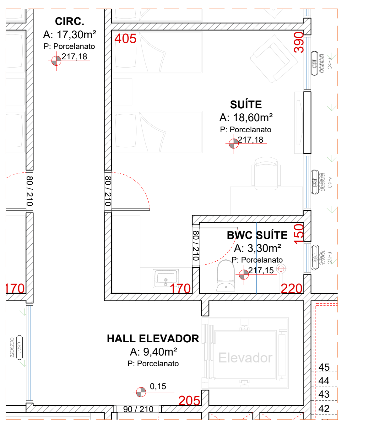
DETALHE 1 - PLANTA BAIXA QUARTO Esc. 1/50
