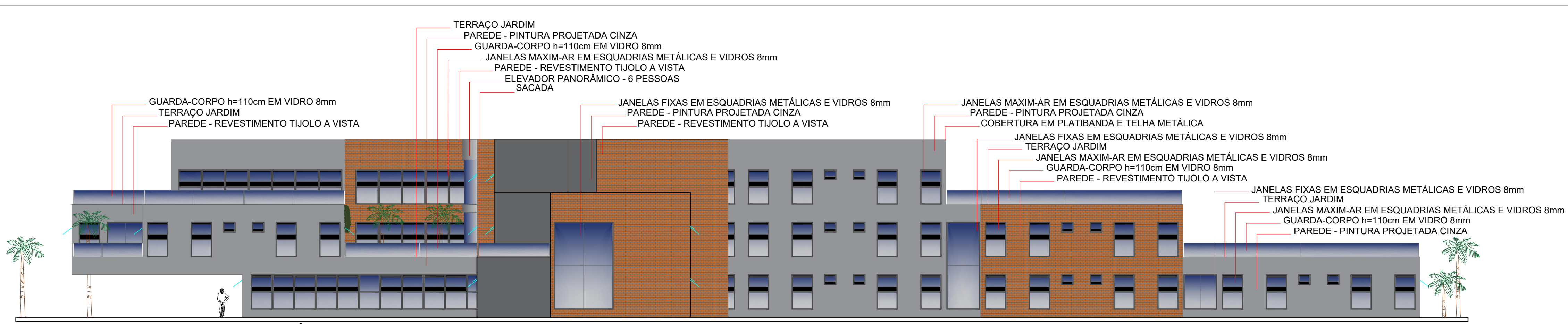
FACHADA SUL - DORMITÓRIOS Esc. 1/150
