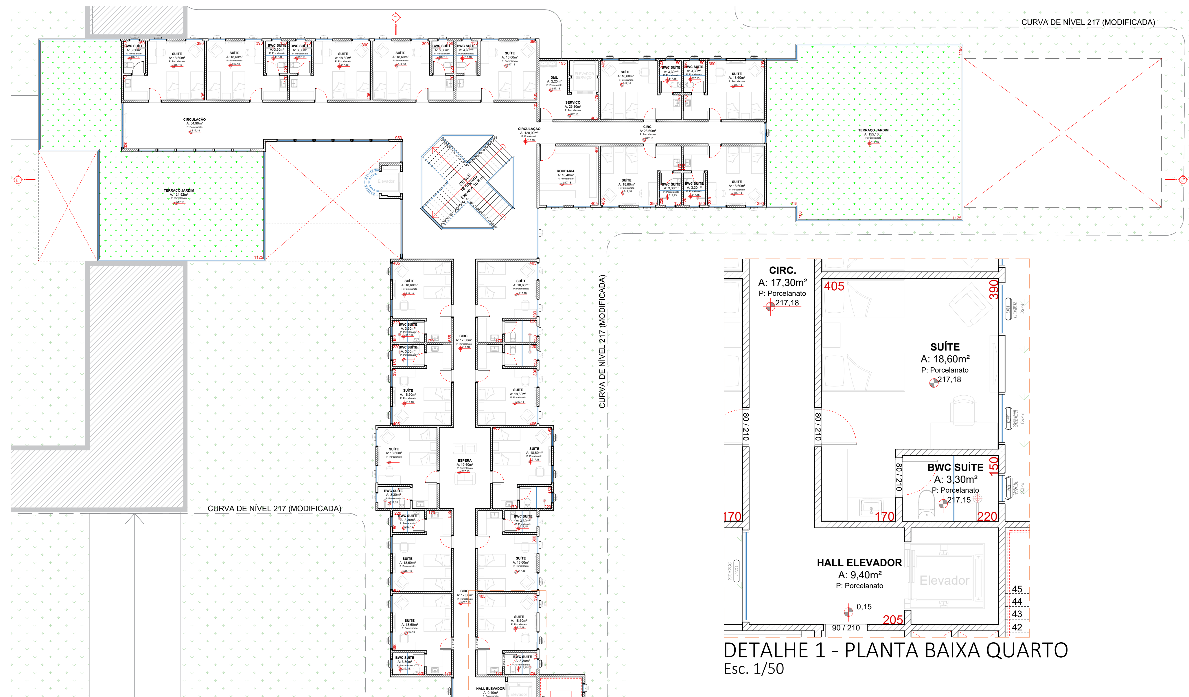
PLANTA BAIXA SETOR DORMITÓRIOS - 2º PAVIMENTO Esc. 1/150
