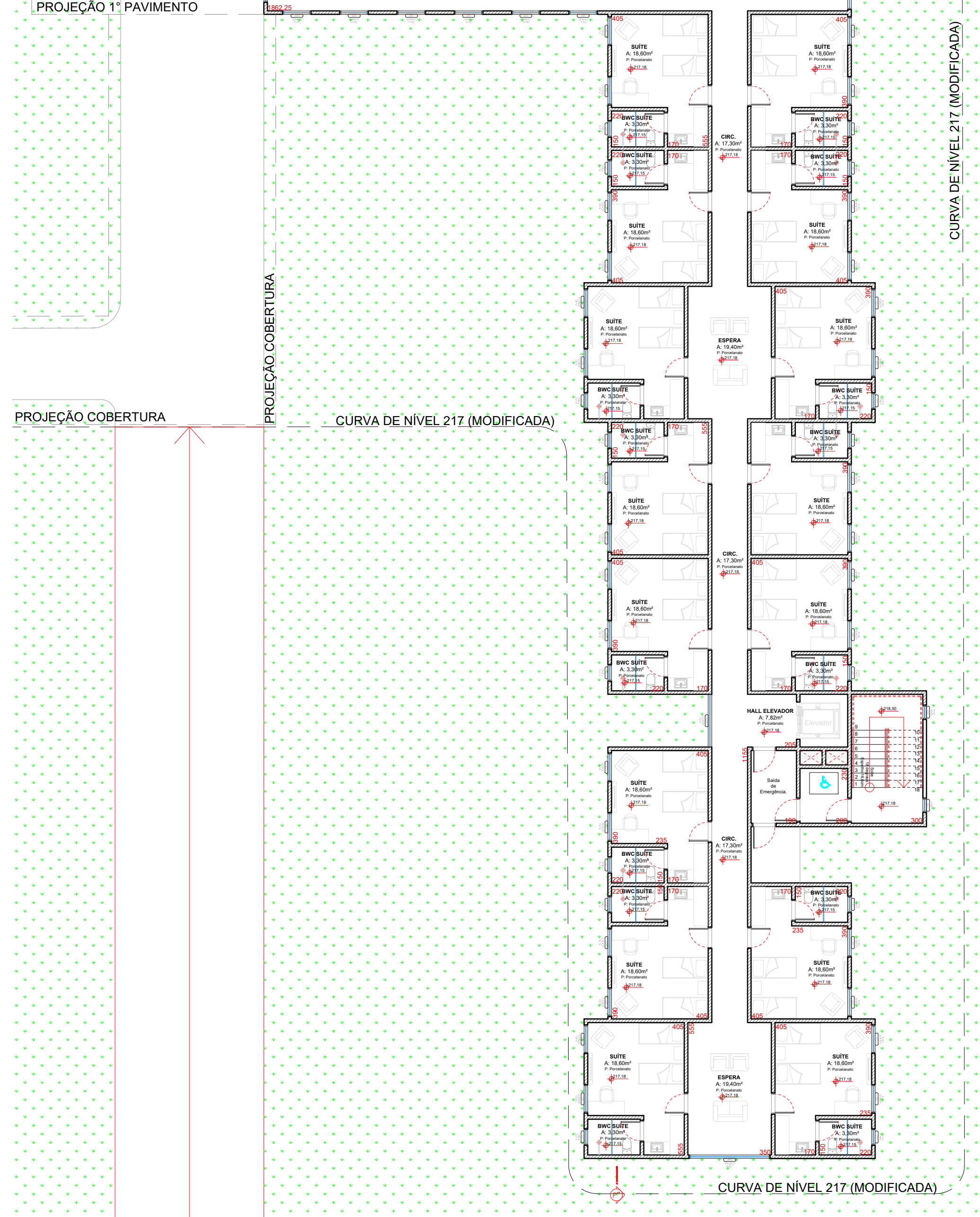
PLANTA BAIXA SETOR DORMITÓRIOS - PAV. TÉRREO Esc. 1/150
