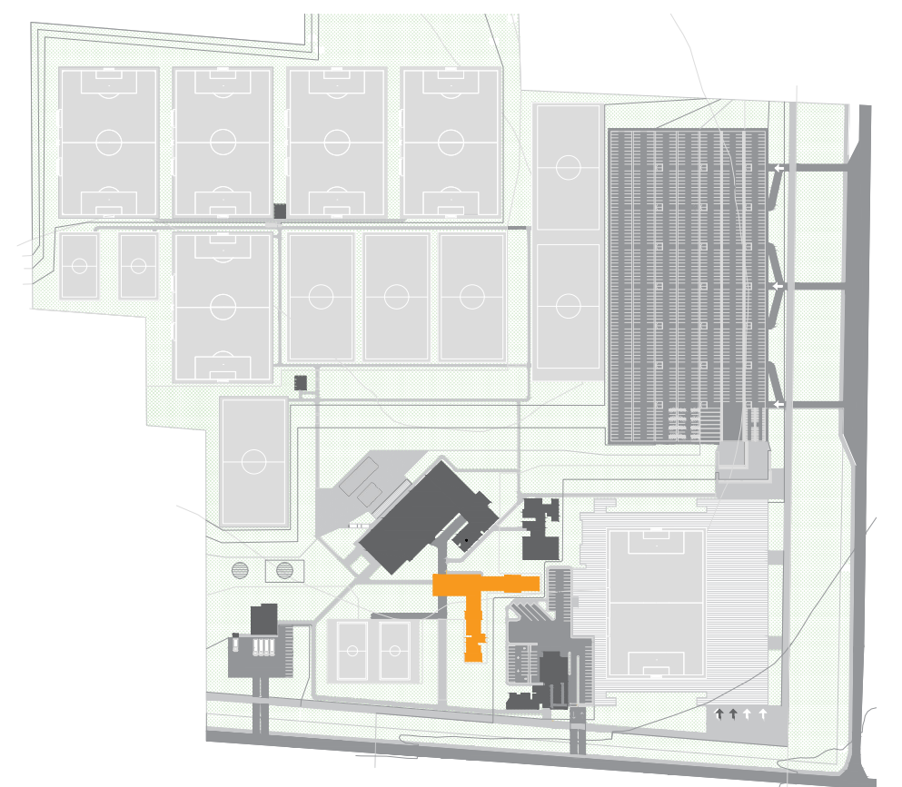
PLANTA DE SITUAÇÃO DORMITÓRIOS Esc. 1/5000
