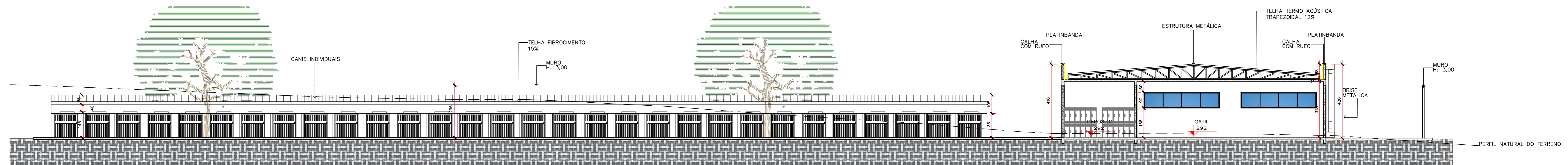
CORTE C6 Escala 1/100
