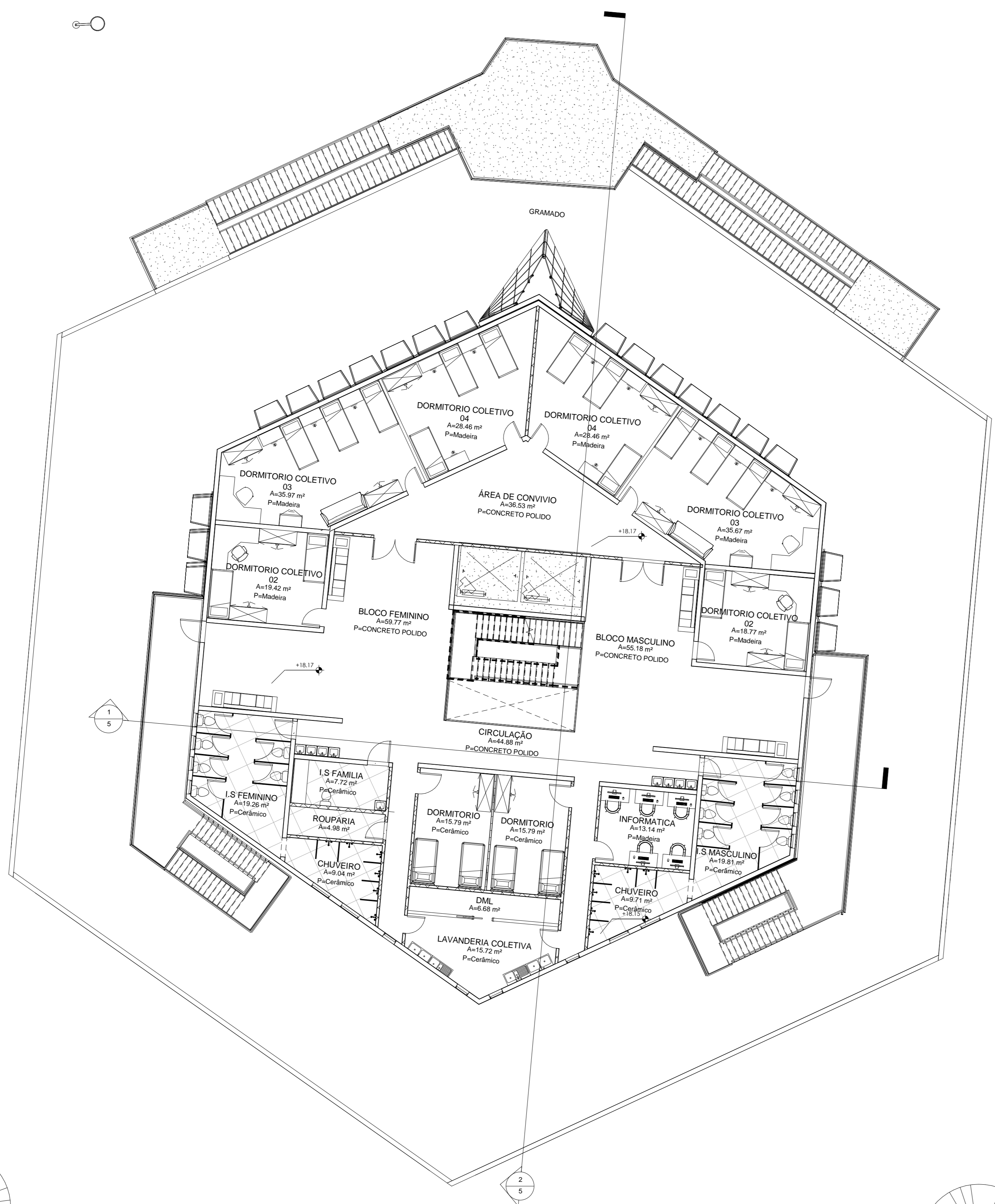
1 QUARTO PAVIMENTO 1 : 100
