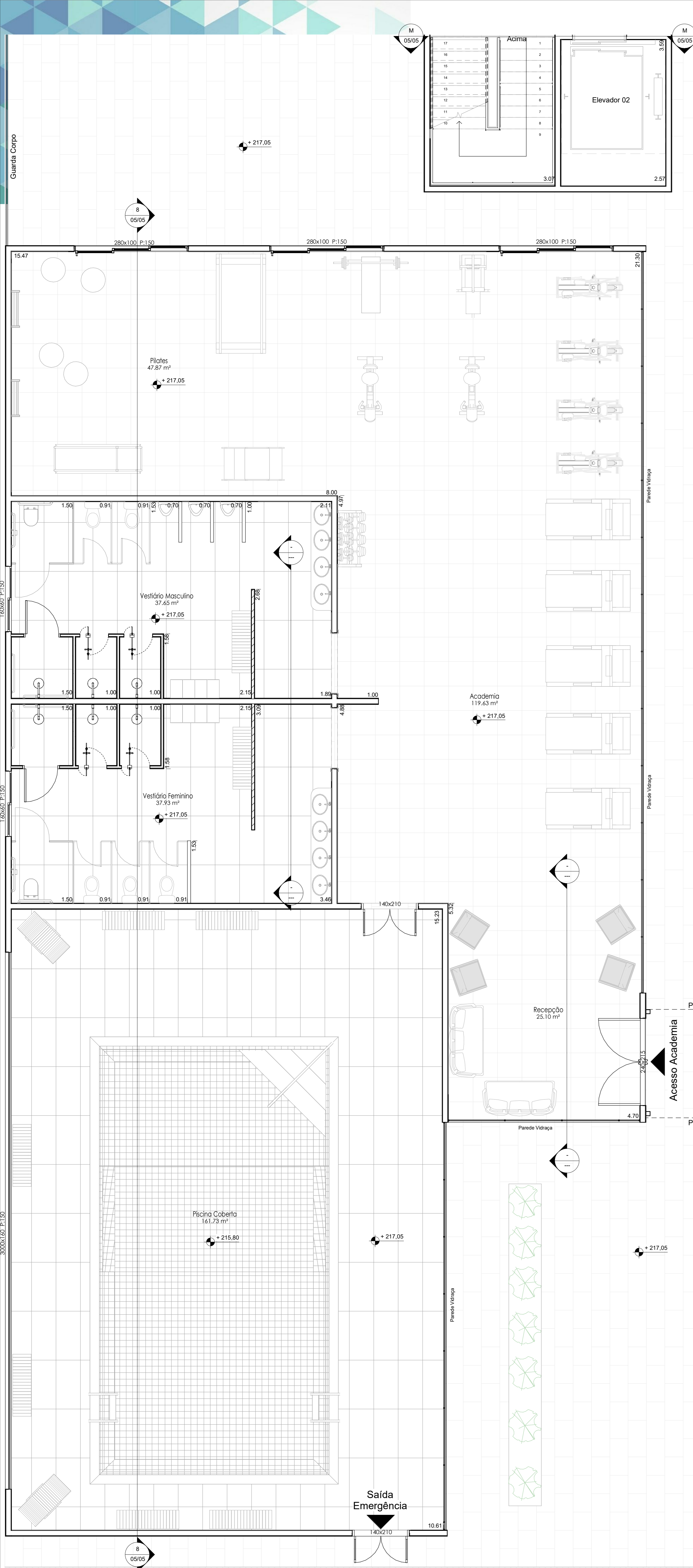
1 Planta Baixa Pav Térreo - Academia 1 : 50
