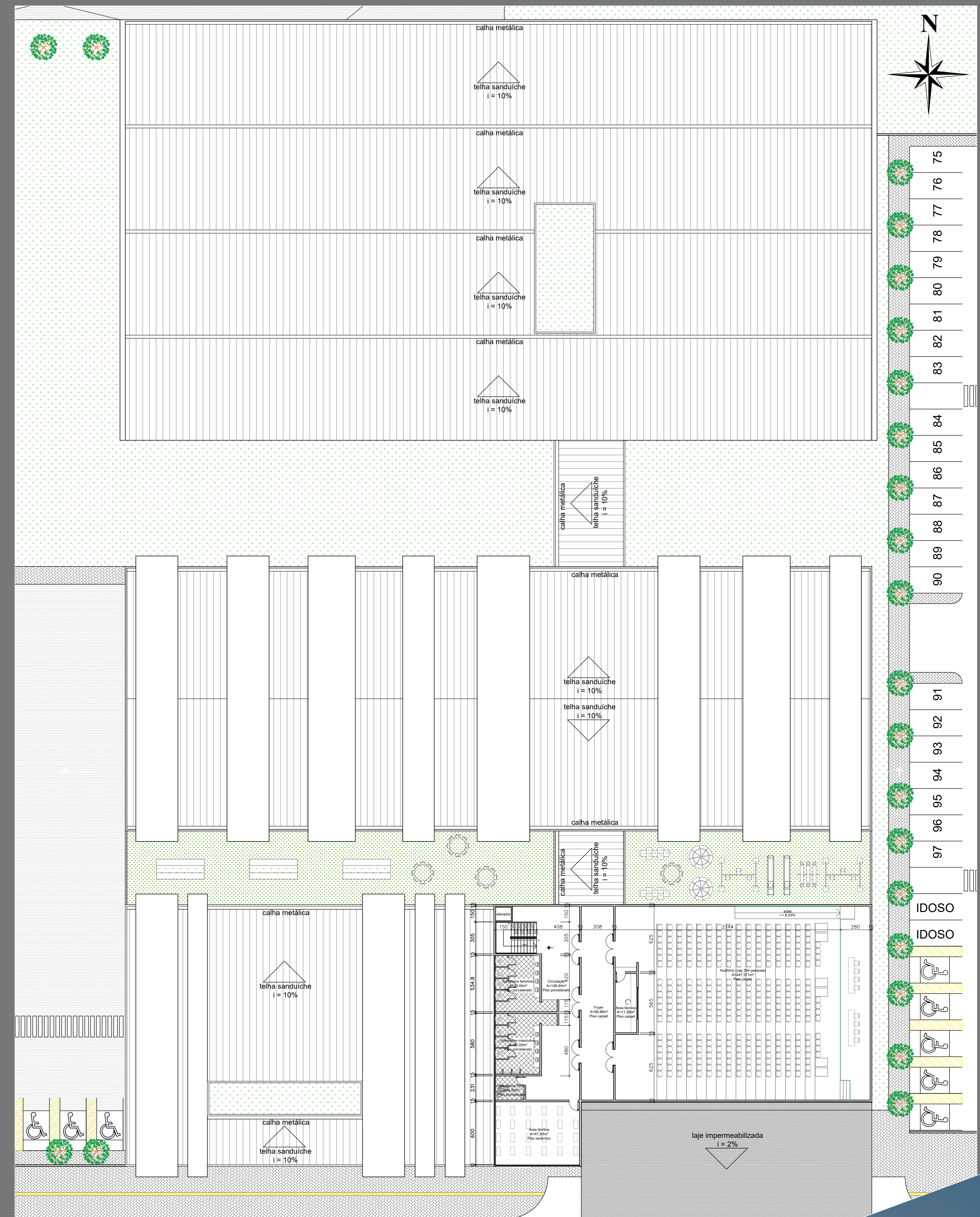
Planta baixa 2º pavimento ESC.: 1/175
