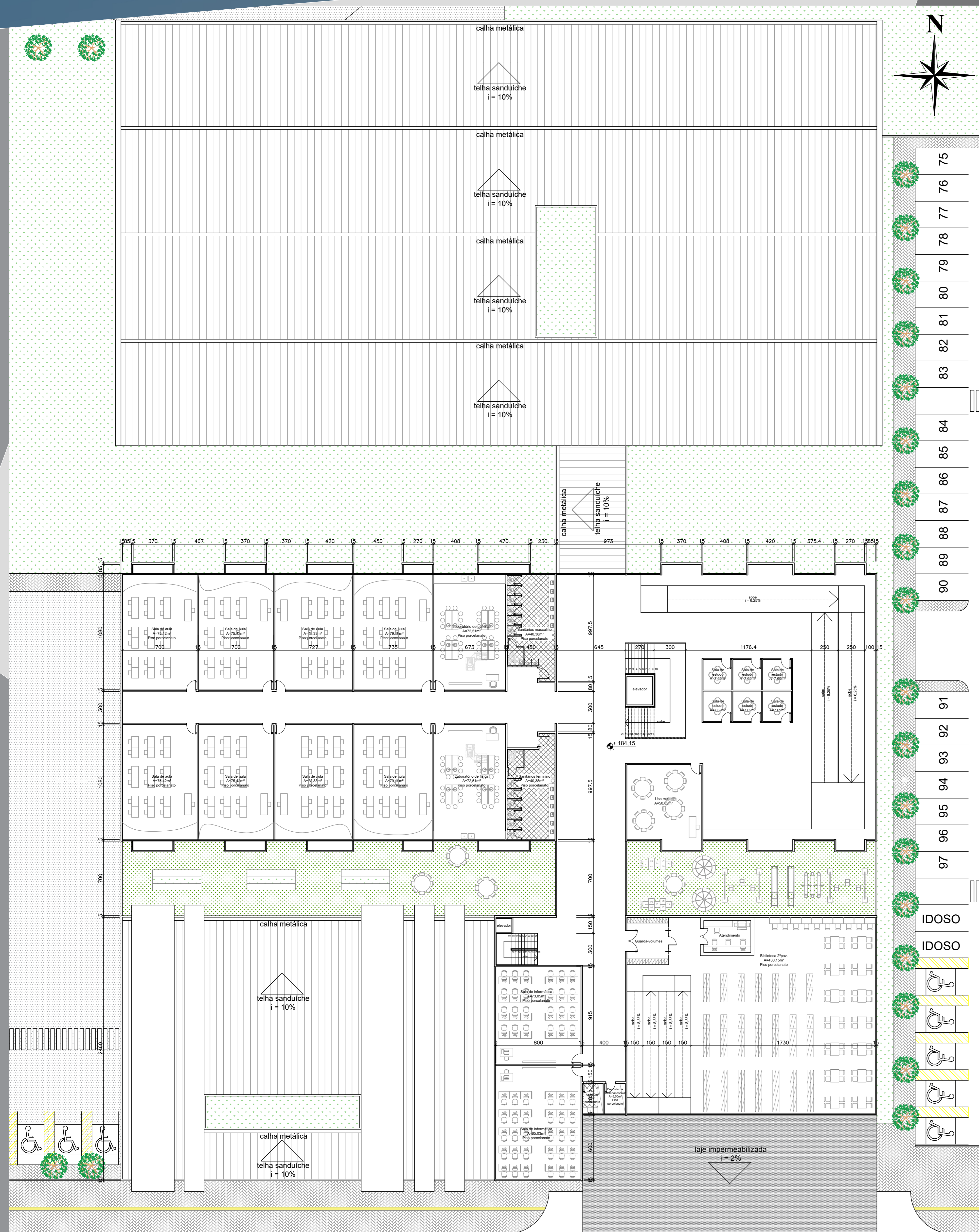
Planta baixa 1º pavimento ESC.: 1/175
