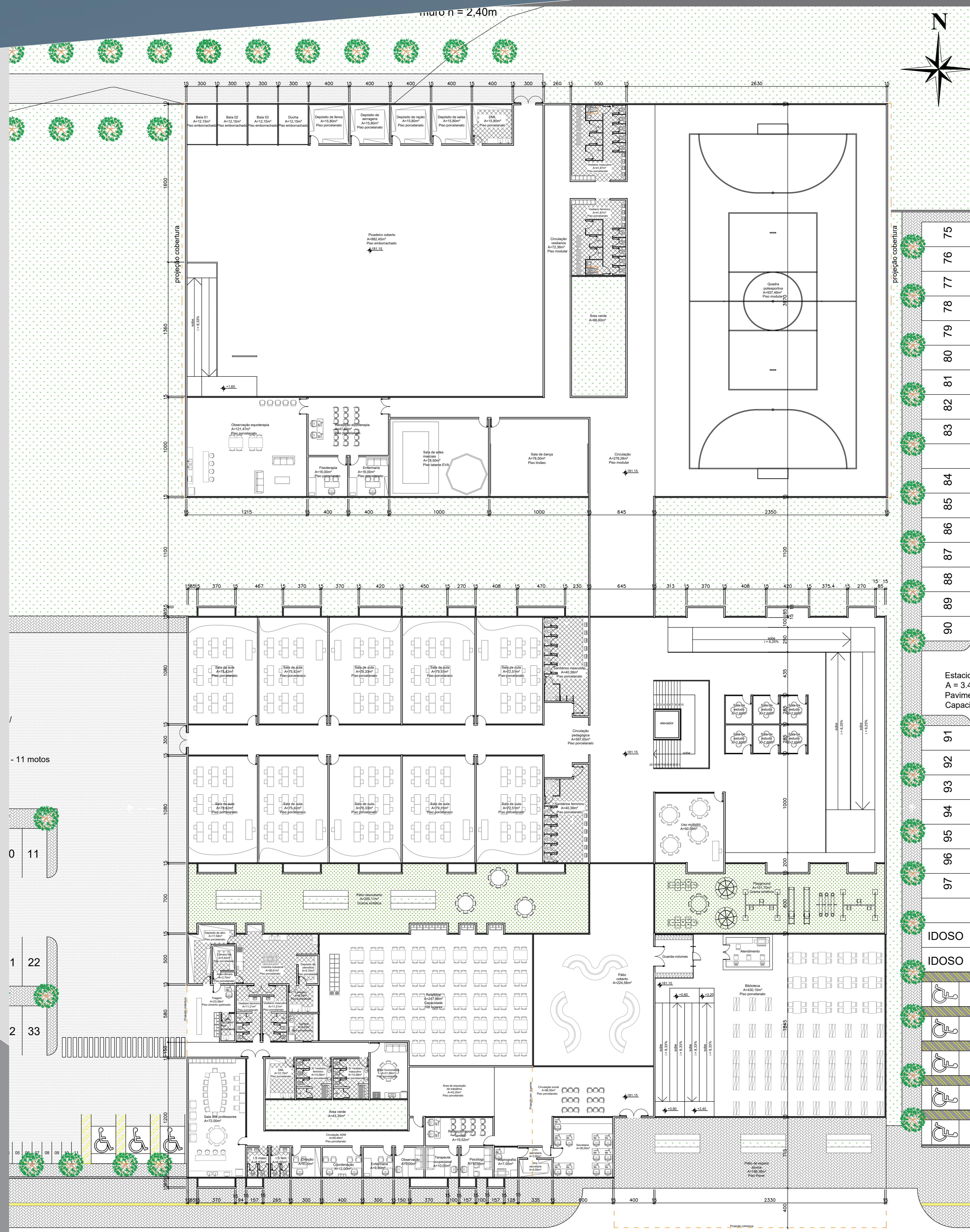
Planta baixa térreo ESC.: 1/175
