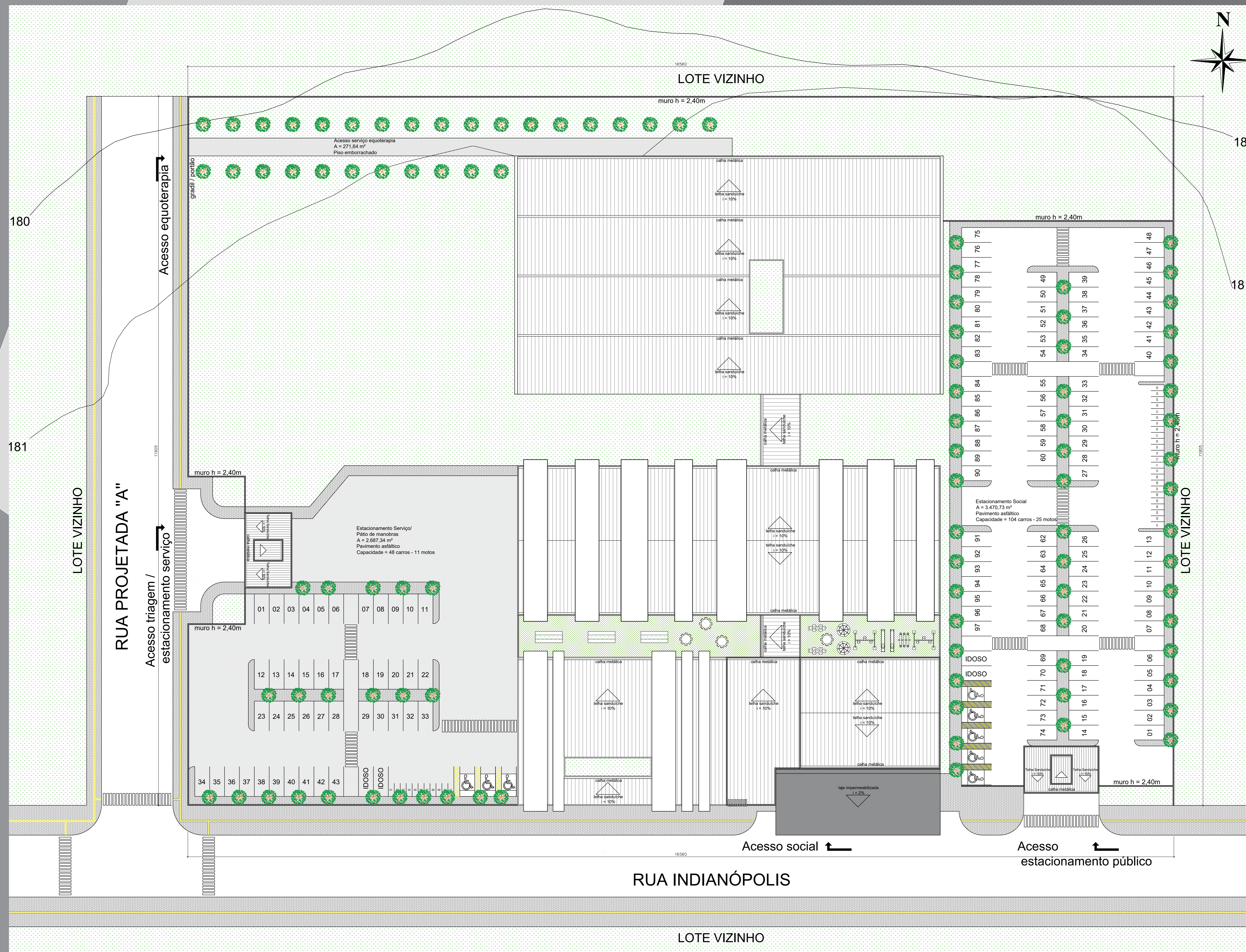
Implantação e cobertura ESC.: 1/250
