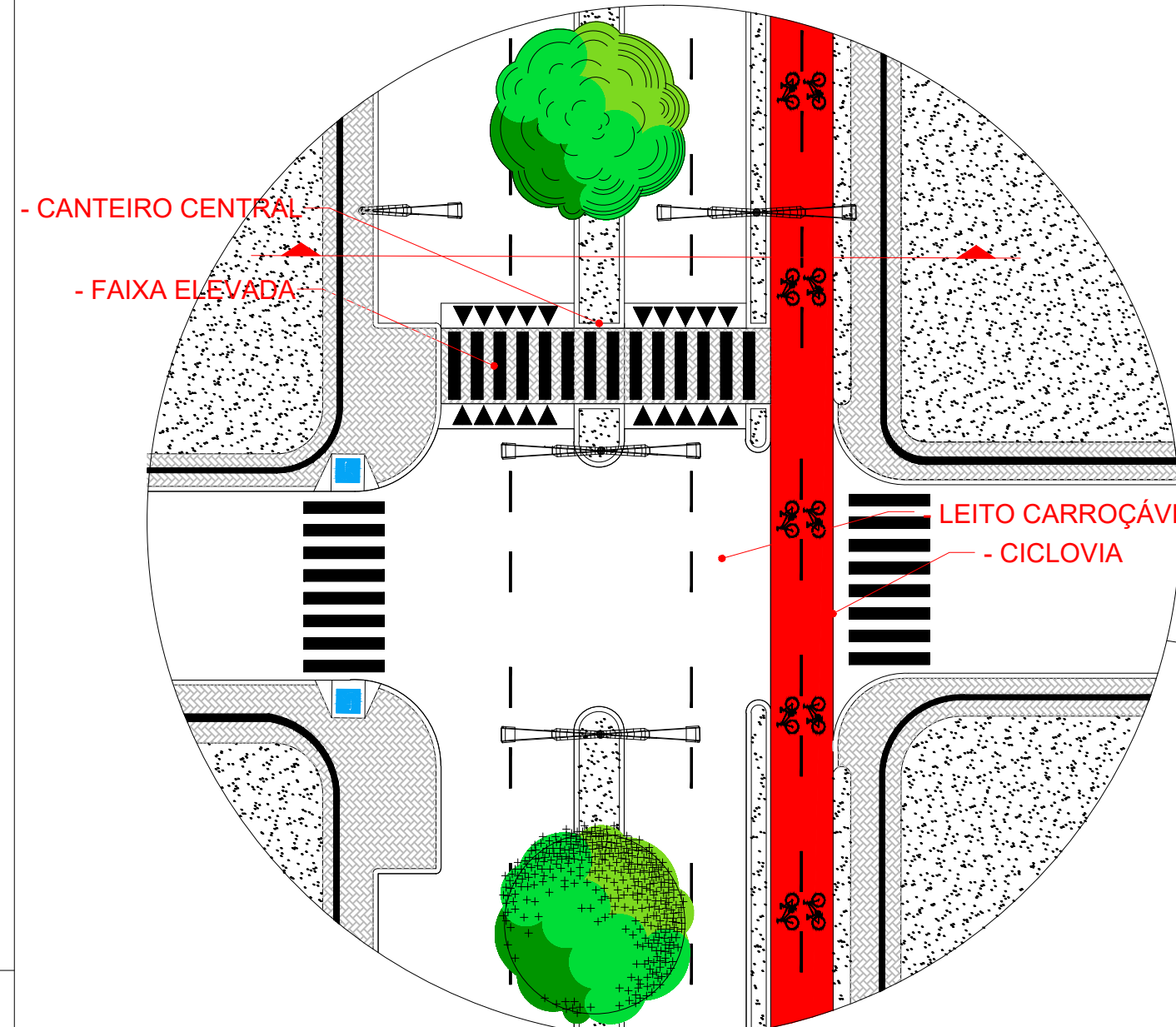
DETALHE AVENIDA DAS ROSAS ESCALA: 1/200
