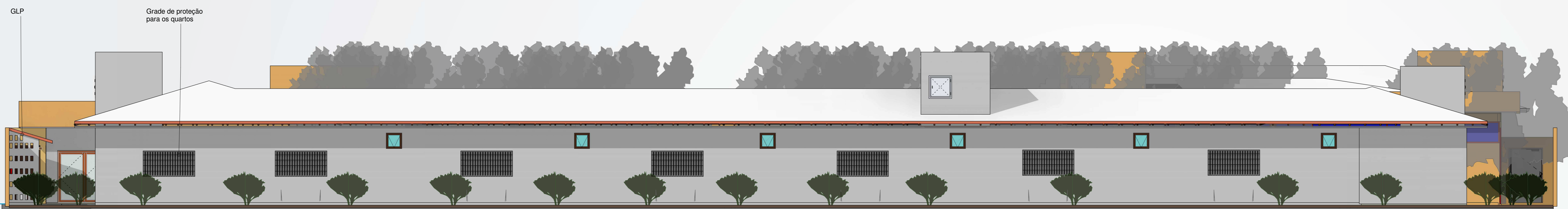
2 Elevação Sul 1:75
