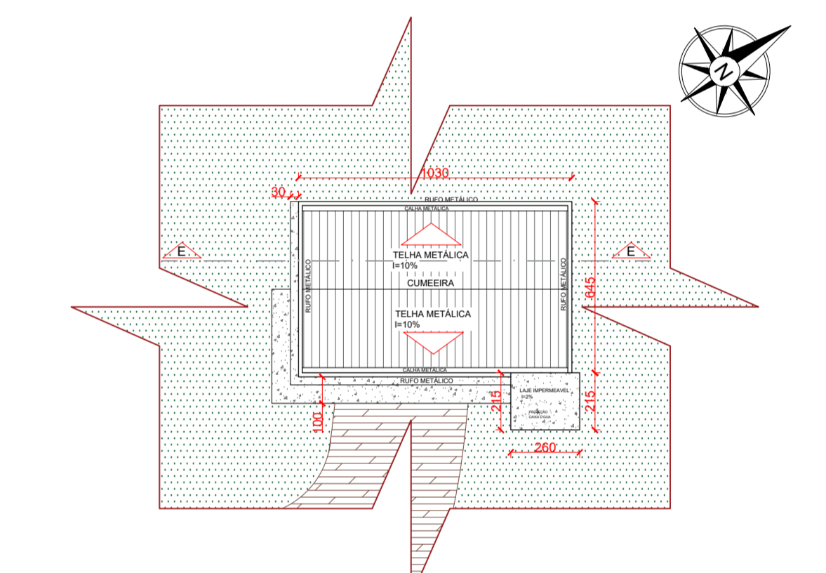
PLANTA DE COBERTURA 1/200
