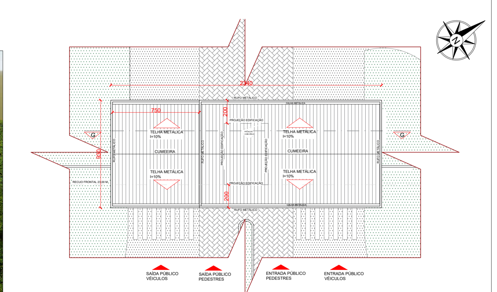
PLANTA DE COBERTURA 1/200
