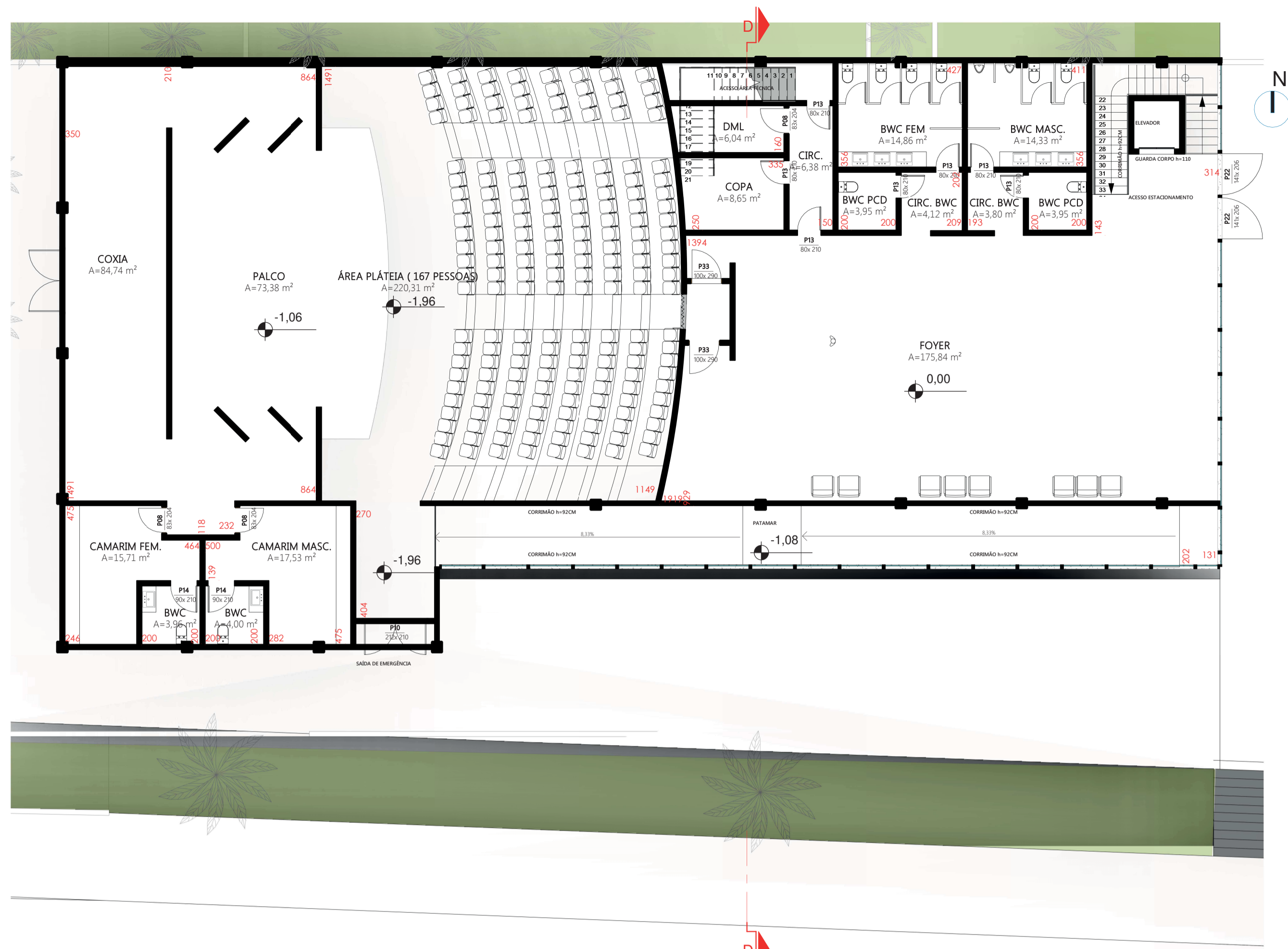
PLANTA BAIXA TERREO AUDITÓRIO 1/125
