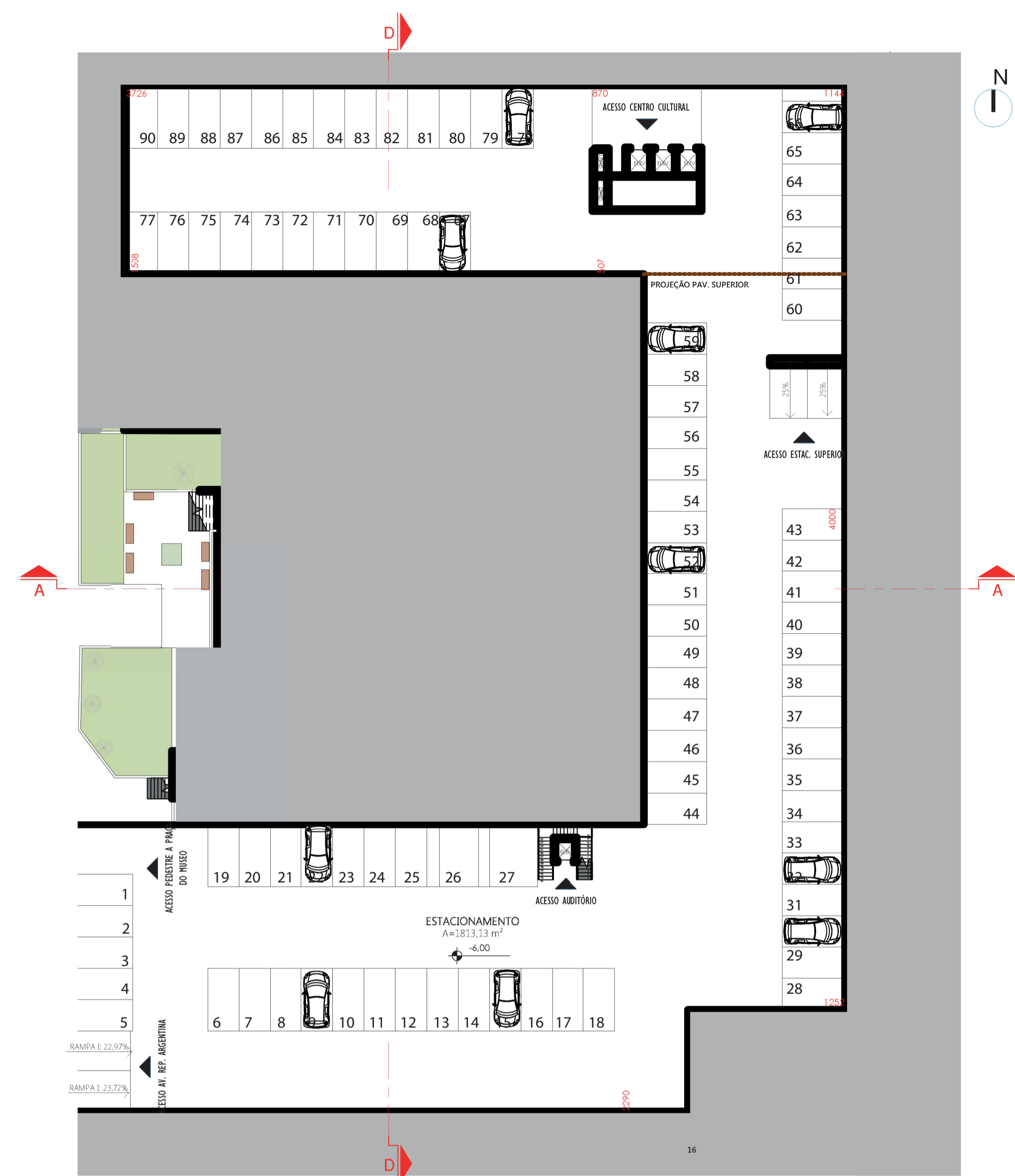
PLANTA BAIXA TERREO ESTACIONAMENTO 1/300
