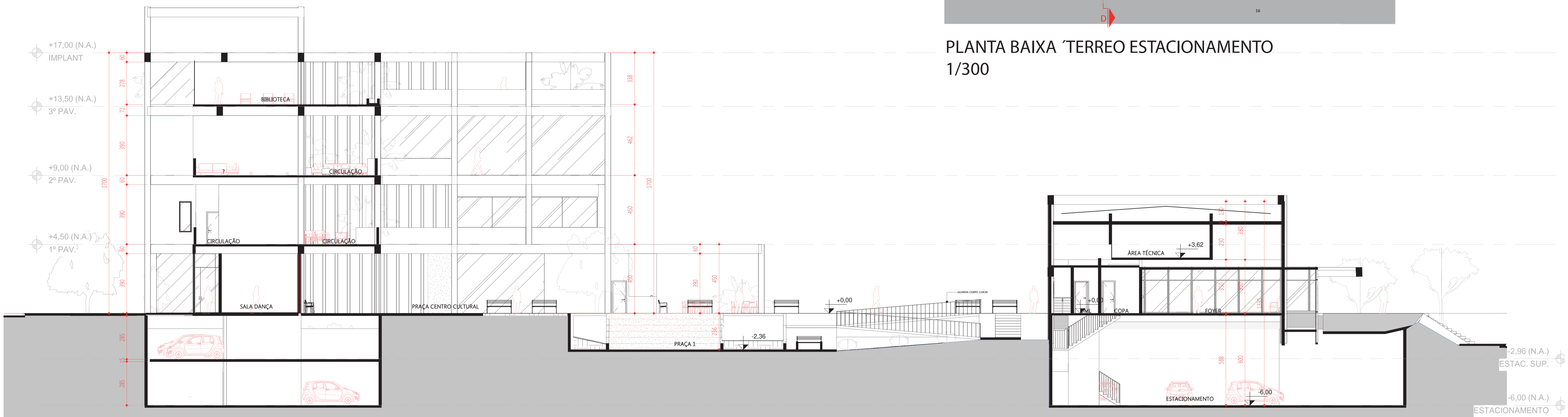
CORTE DD 1/125
