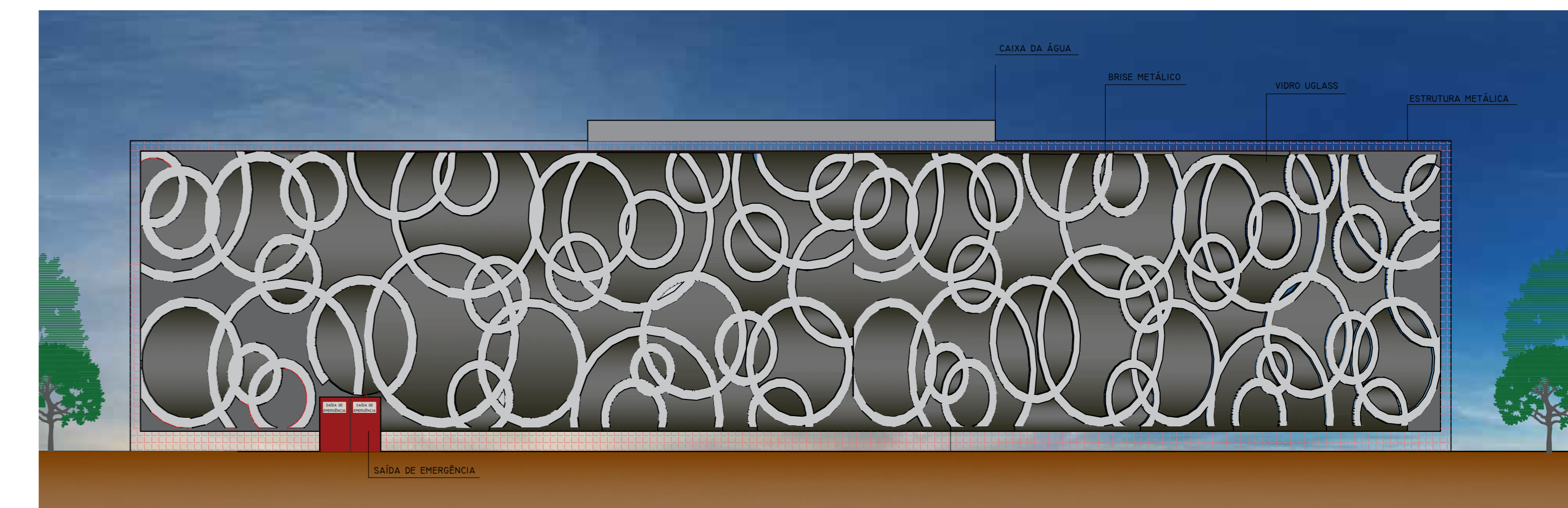
FACHADA NOROESTE ESC:1/200
