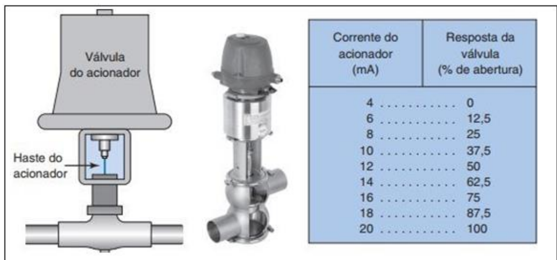
Figure 2: Funcionamento de uma válvula de controle proporcional.
